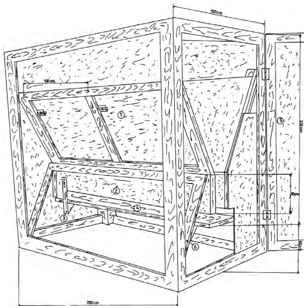
Schia 11. Instalație de contenție pentru cerb comun.
