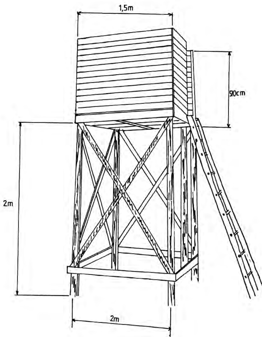
Schița 12. Hochstand „la înălțime”.
