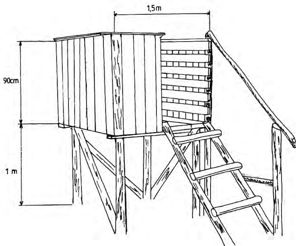
Schița 13. Hochstand „semiînălțime”.
