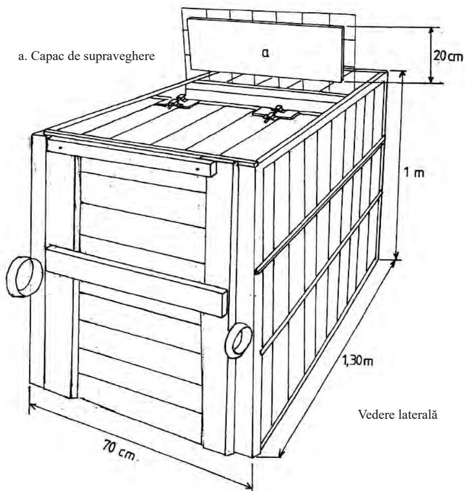
Schița 4m. Ladă transport mistreți.
