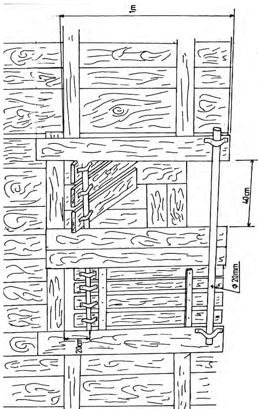
Schița 13m. Poartă capcană dublă.
