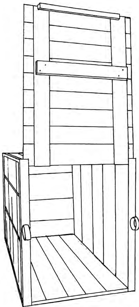
Schița 5m. Ladă transport mistreți.
