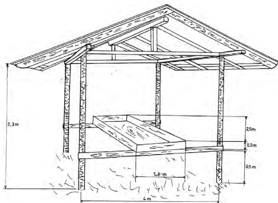
Schița 3. Hrănitore ce cervide - furaj concentrat.
