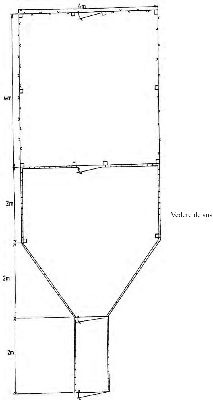
Schița 9m. Capcană dublă.
