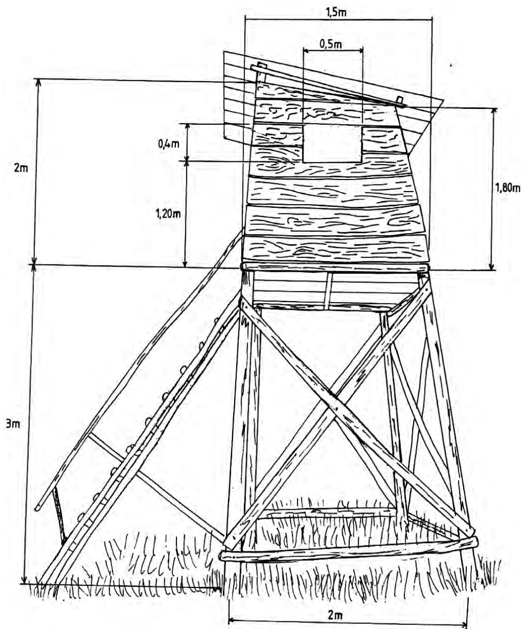
Schița 8. Observator închis.
