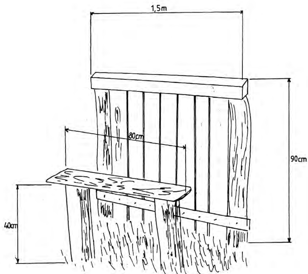
Schița 14m. Stand „pe sol”.
