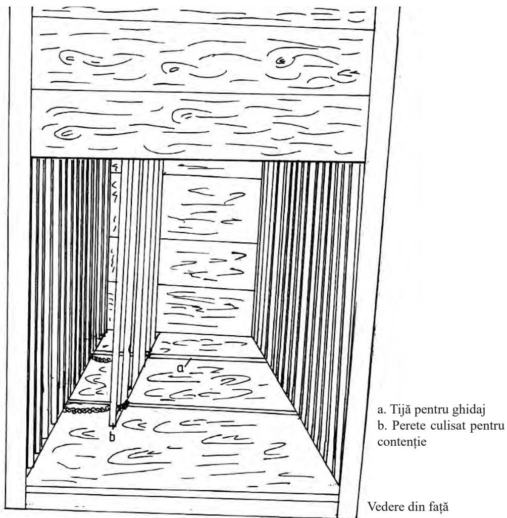
Schița 8m. Ladă conținție.
